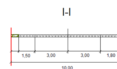
Креслення поперечних профілів М 1:200
